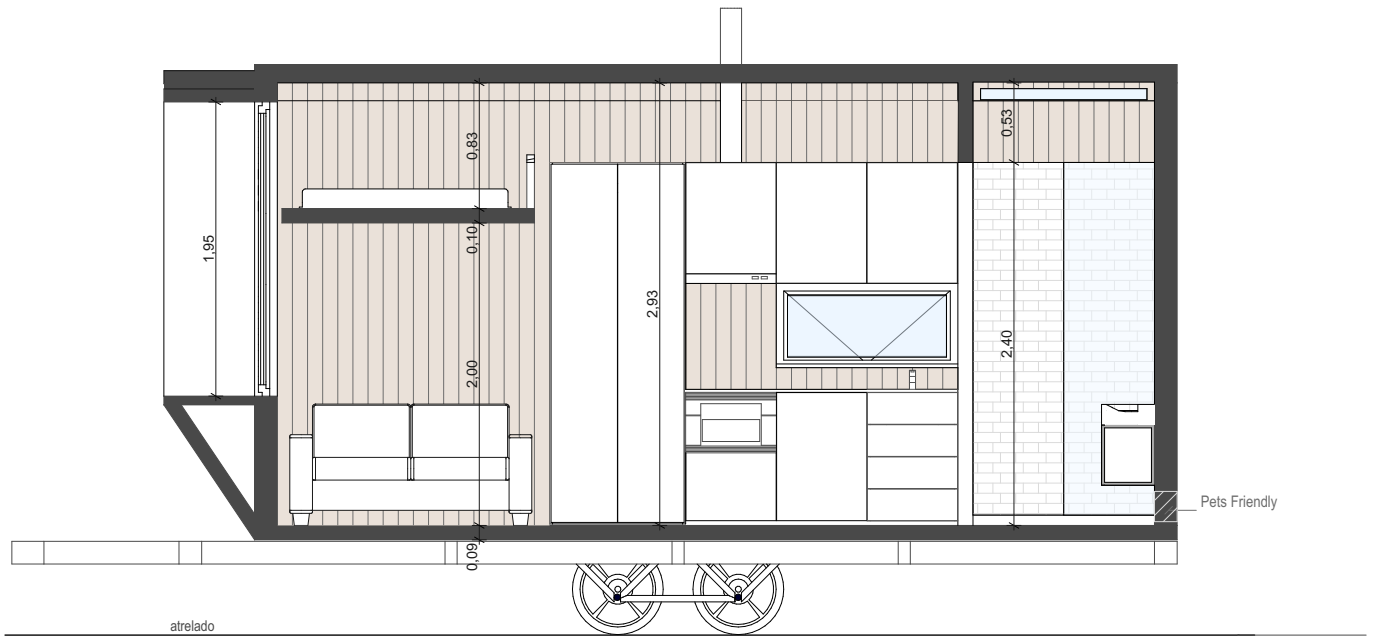
CORTE BB'
