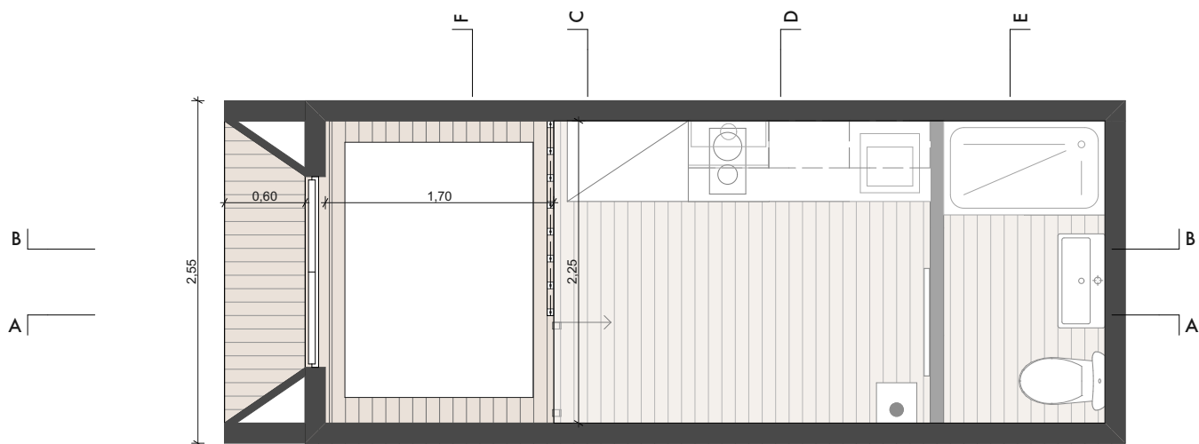
PLANTA MEZZANINOS
