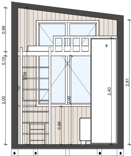
CORTE CC'
