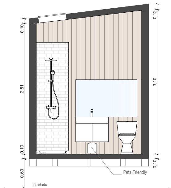
CORTE EE
