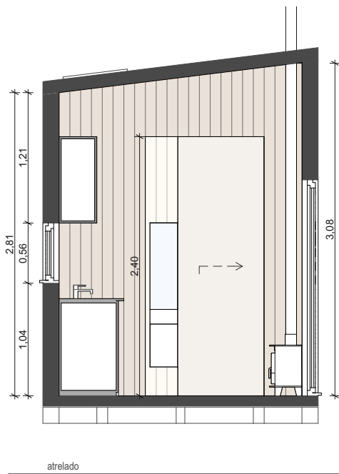
CORTE DD
