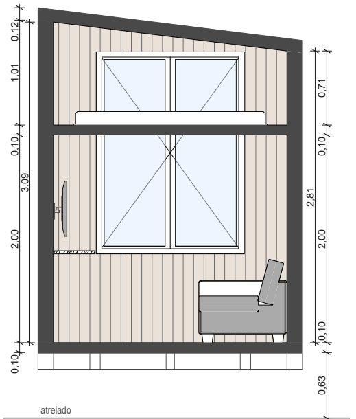
CORTE FF'
