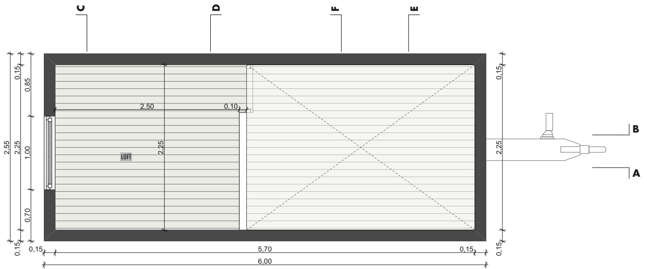
PLANTA LOFT
