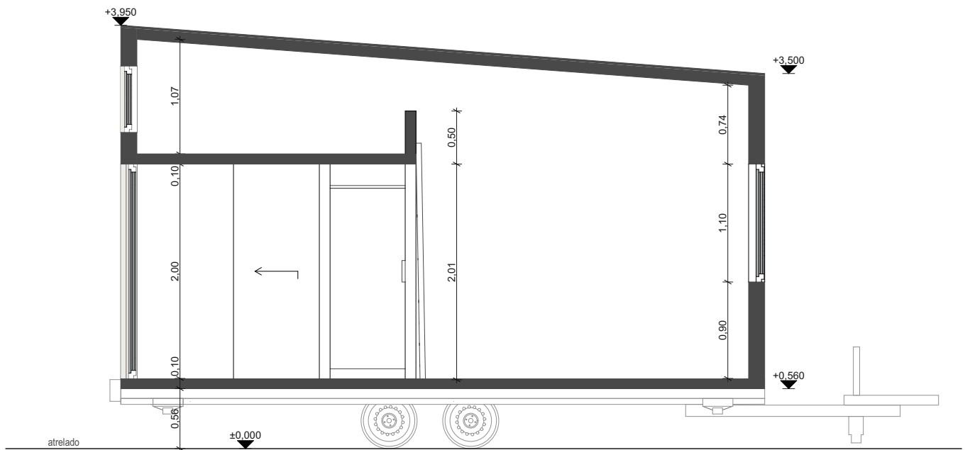
CORTE BB'
