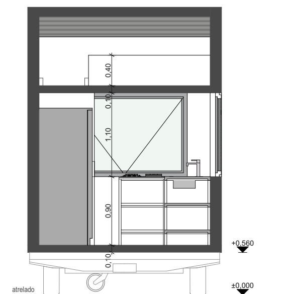
CORTE DD'
