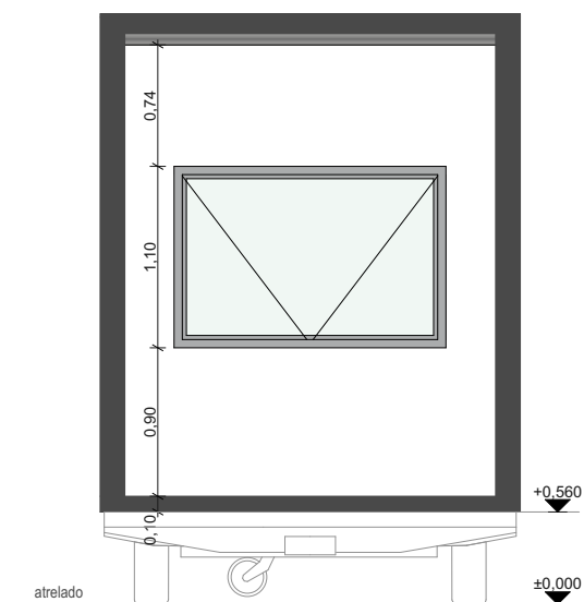
CORTE EE'
